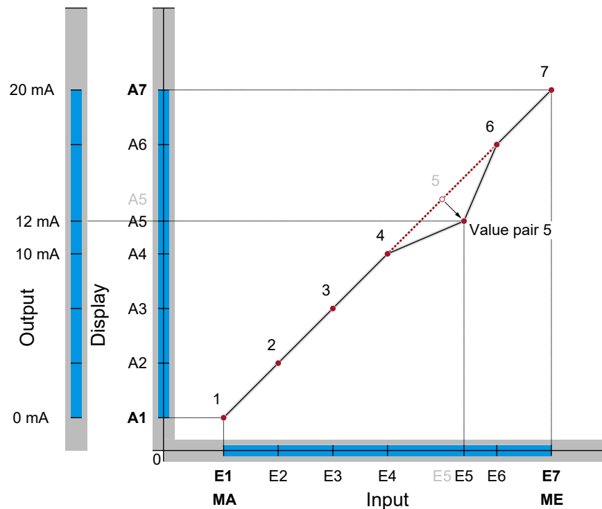
Fig. 86: Table function
