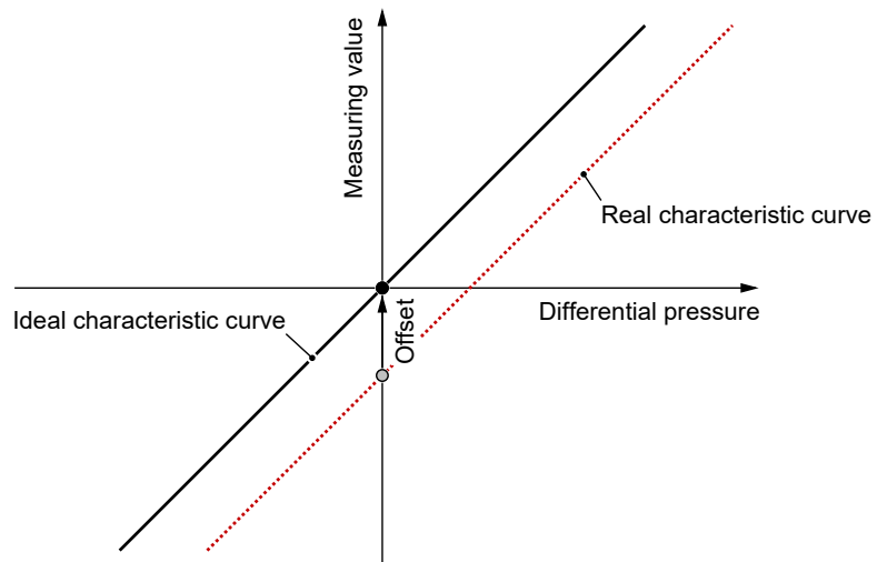
Fig. 79: Offset error
