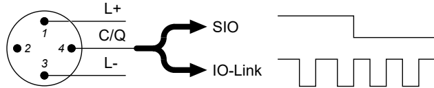
Fig. 38: IO-Link
