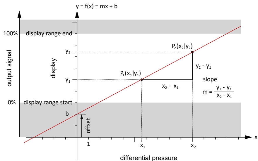
Fig. 94: Linear function
