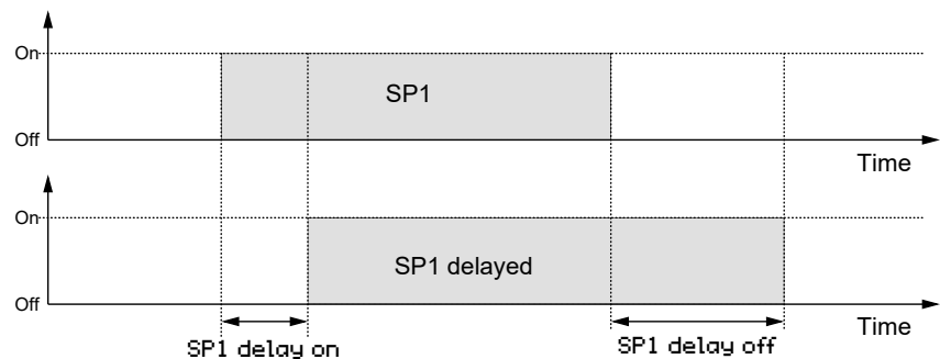
Fig. 131: Delay
