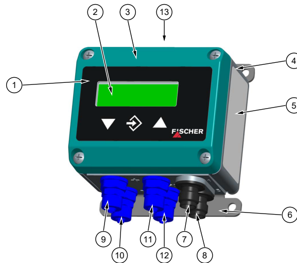
Abb. 3: DE44_LCD Übersicht
