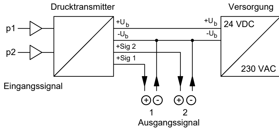
Abb. 6: 3L Anschluss
