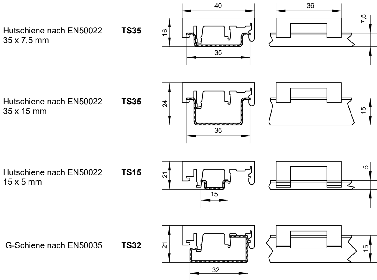
Abb. 29: Maßbild Tragschienenmontage
