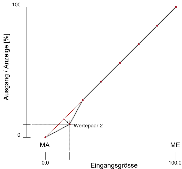
Abb. 18: Tabellenfunktion (Beispiel)
