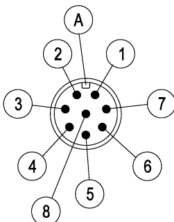
Abb. 24: M12 Stecker 8pol
