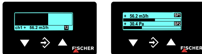
Abb. 10: LC Anzeige (2 Schaltausgänge)
