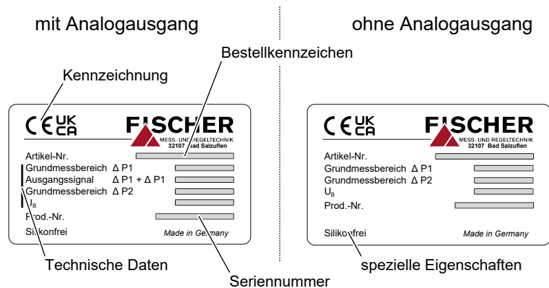
Abb. 4: Typenschild
