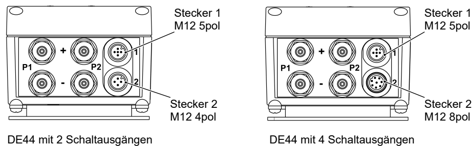
DE44 mit 2 Schaltausgängen
