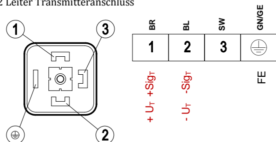
2 Leiter Transmitteranschluss
