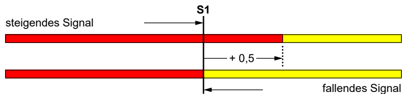
Abb. 79: Beispiel: Hysterese S1
