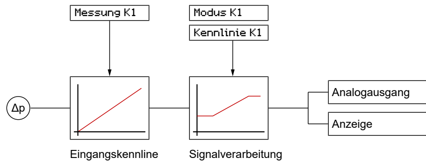
Abb. 45: Parametrierung der Kennlinie K1
